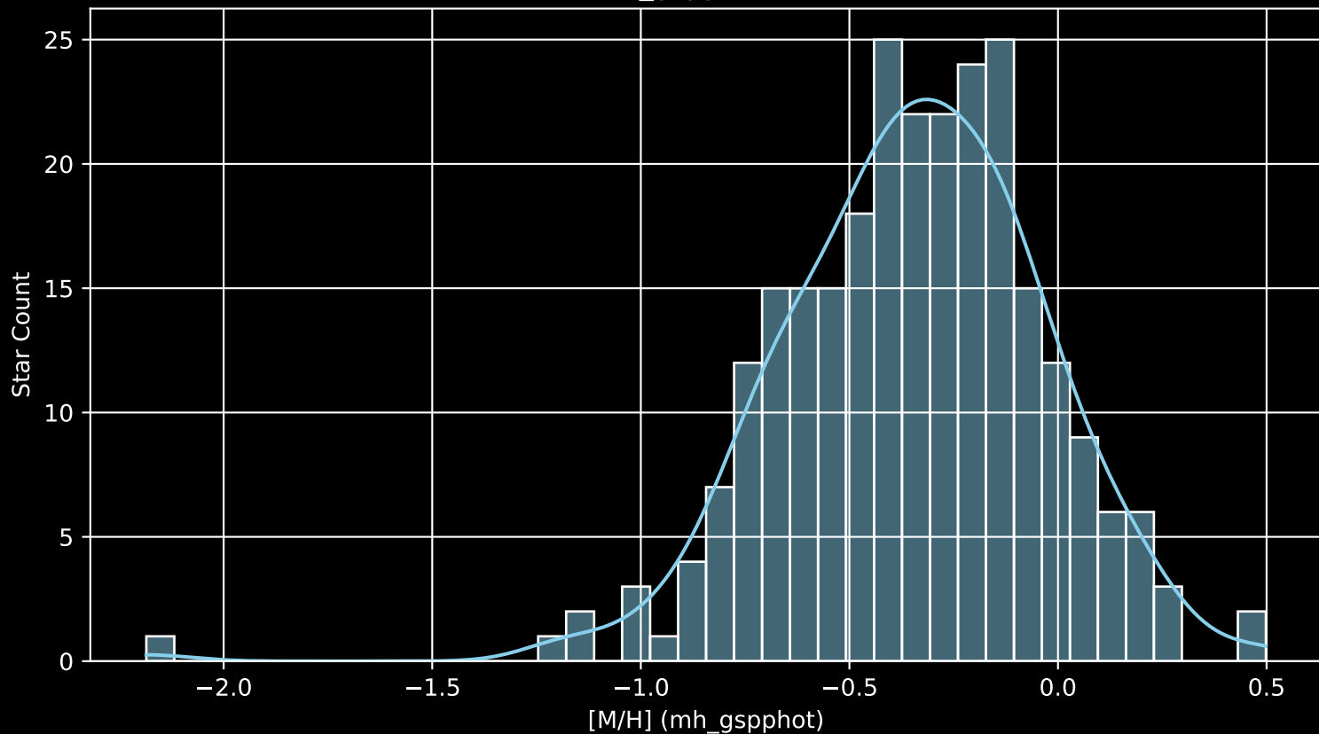
GALAH DR4 Field: [501] [M/H] (mh_gspphot) (n= 265)
