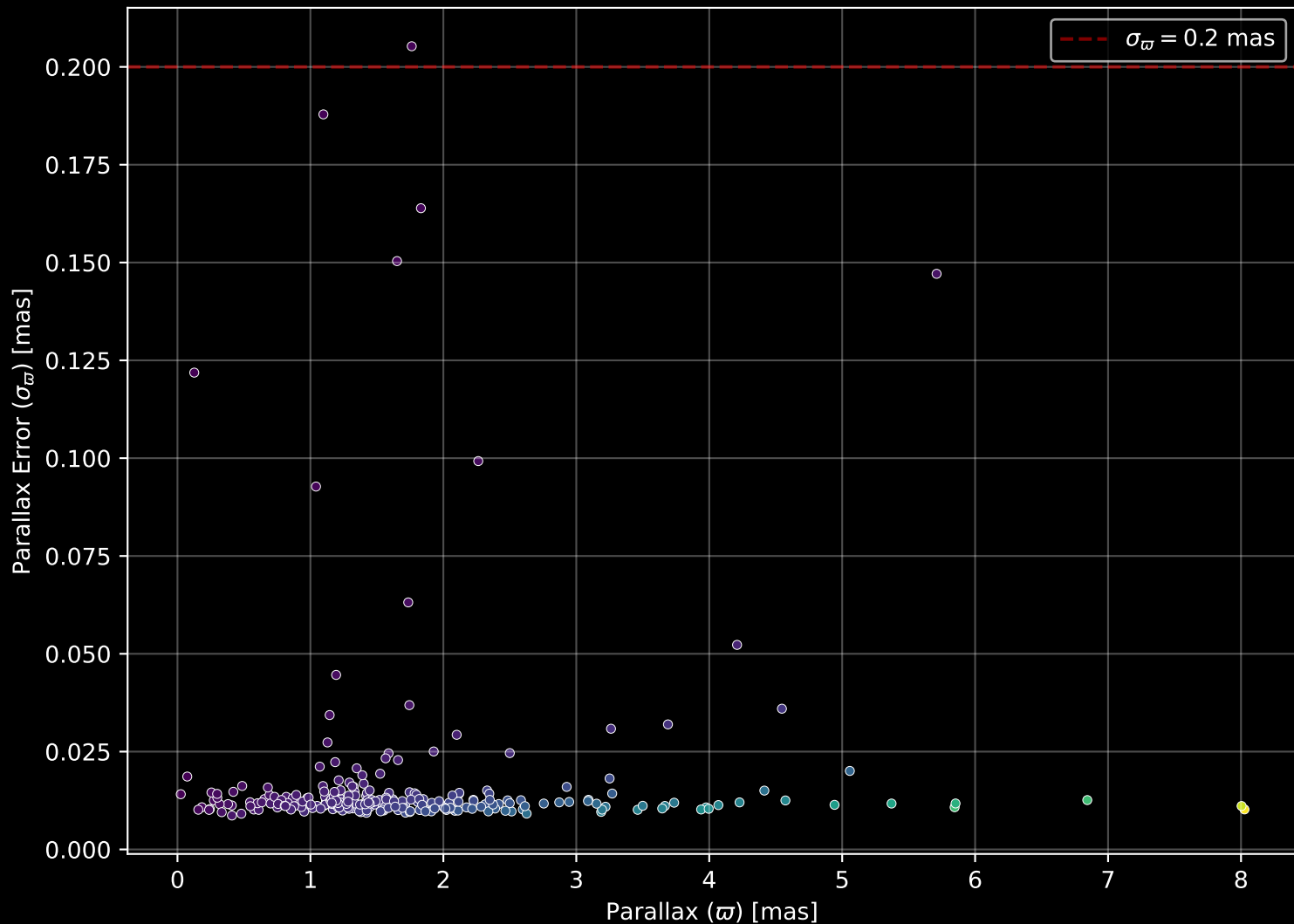
GALAH DR4 Field: [501] Parallax Quality (n= 266)
