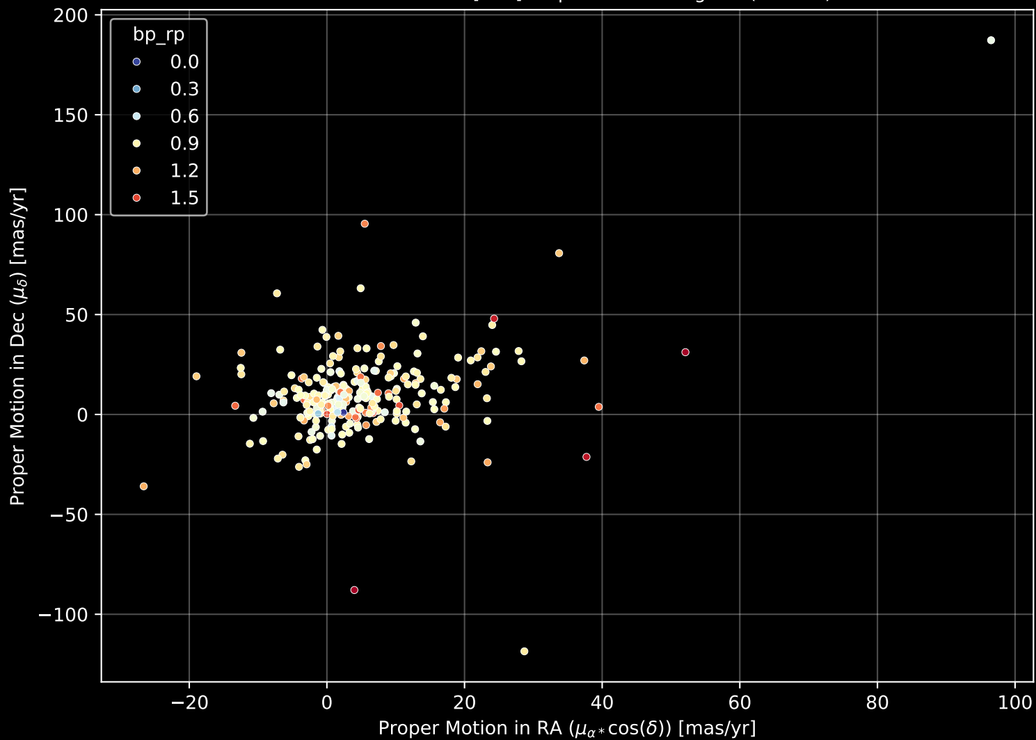
GALAH DR4 Field: [501] Proper Motion Diagram (n= 266)
