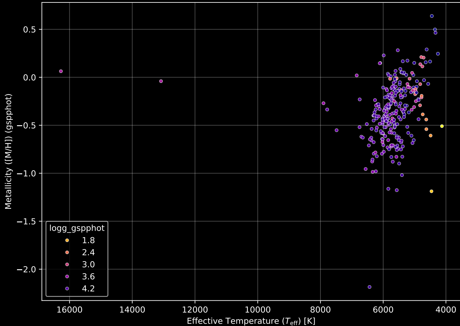
GALAH DR4 Field: [501] Stellar Population Parameters (n= 266)
